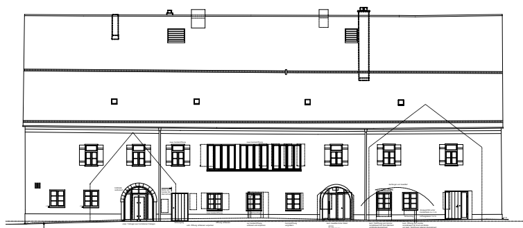
Hofseite West
